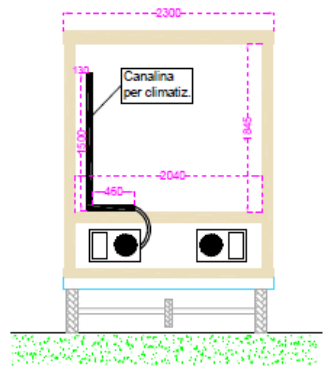
PROSPETTO LATERALE DESTRO
