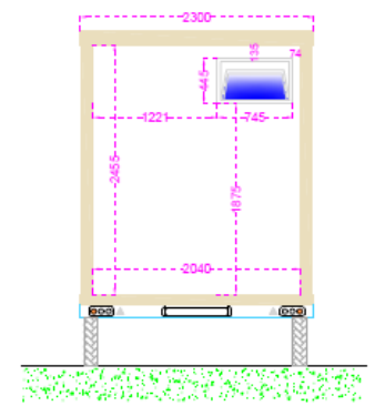
PROSPETTO LATERALE SINISTRO
