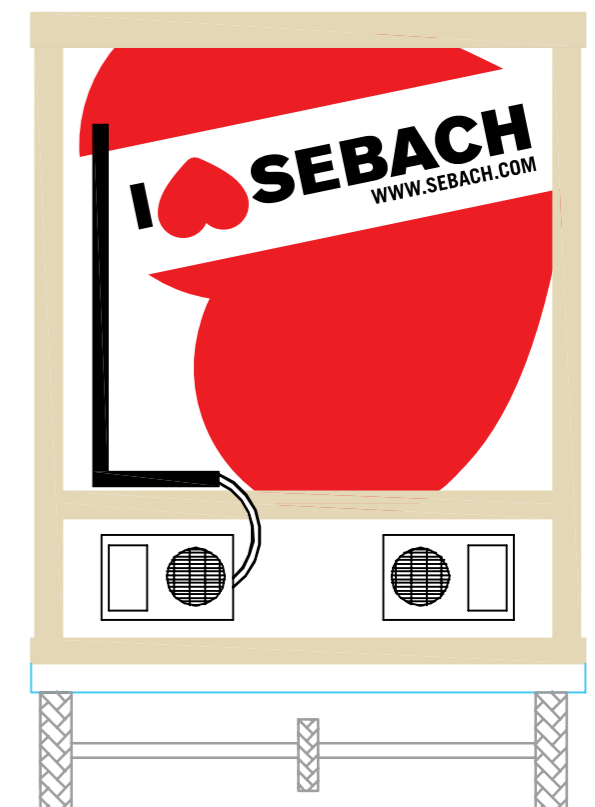
PROSPETTO LATERALE DESTRO
